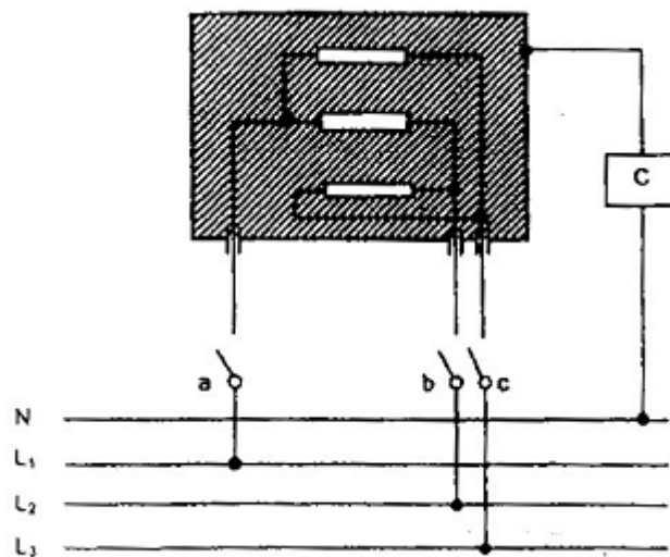
Hình 3 - Sơ đồ mạch điện để đo dòng điện rò ở nhiệt độ làm việc đối với đầu nối ba pha của thiết bị cấp II
