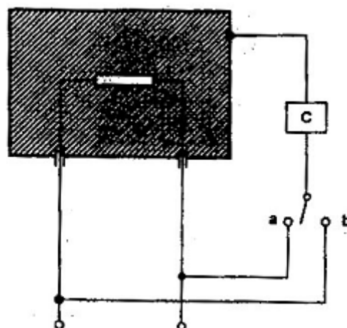
Hình 1 - Sơ đồ mạch điện để đo dòng điện rò ở nhiệt độ làm việc đối với đầu nối một pha của thiết bị cấp II
