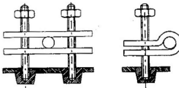
Hình 8 - Thiết bị thử nghiệm uốn
